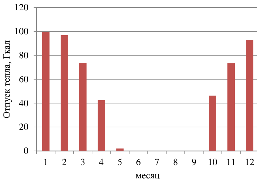
Рисунок 1.4 – Оптимальный температурный график отпуски тепловой энергии для центральной котельной с. Новодостовалово
