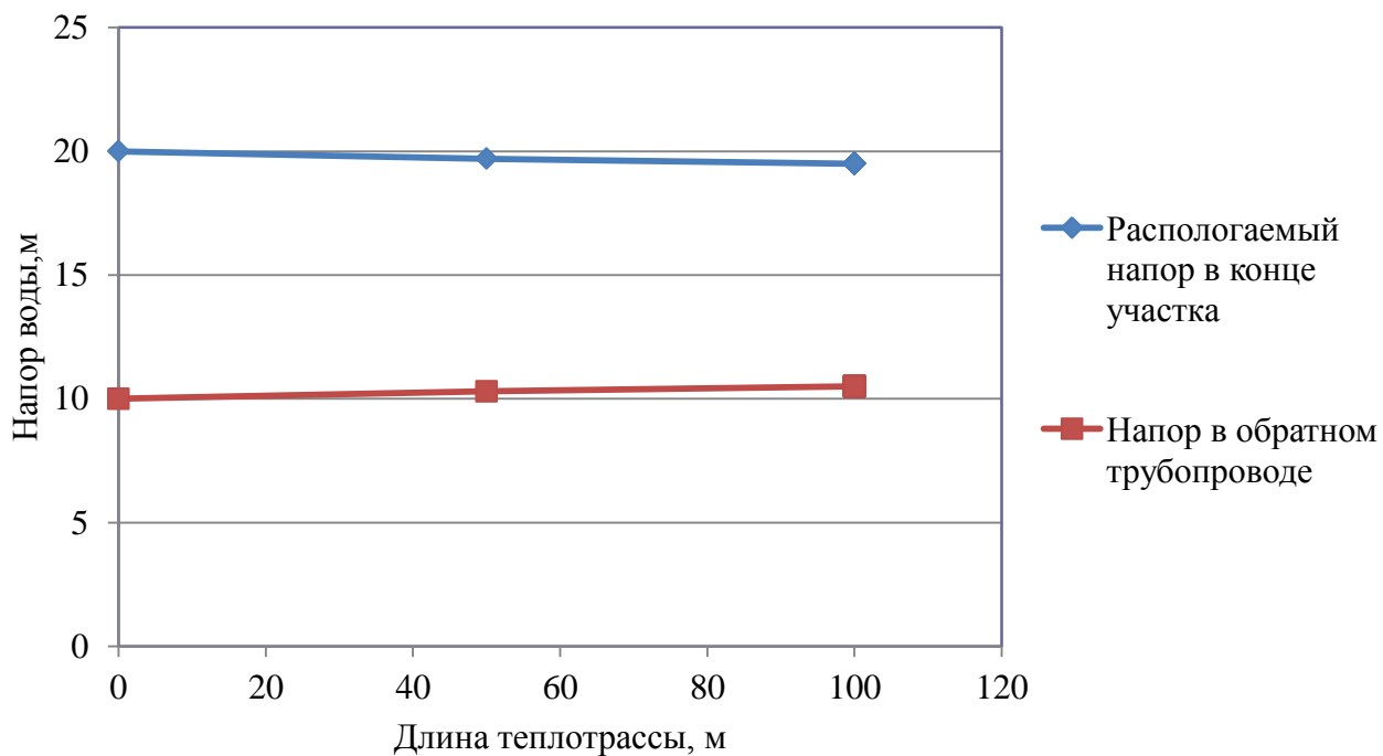
Рисунок 2.6 – Пьезометрический график тепловой сети школьной котельной с. Романовское
