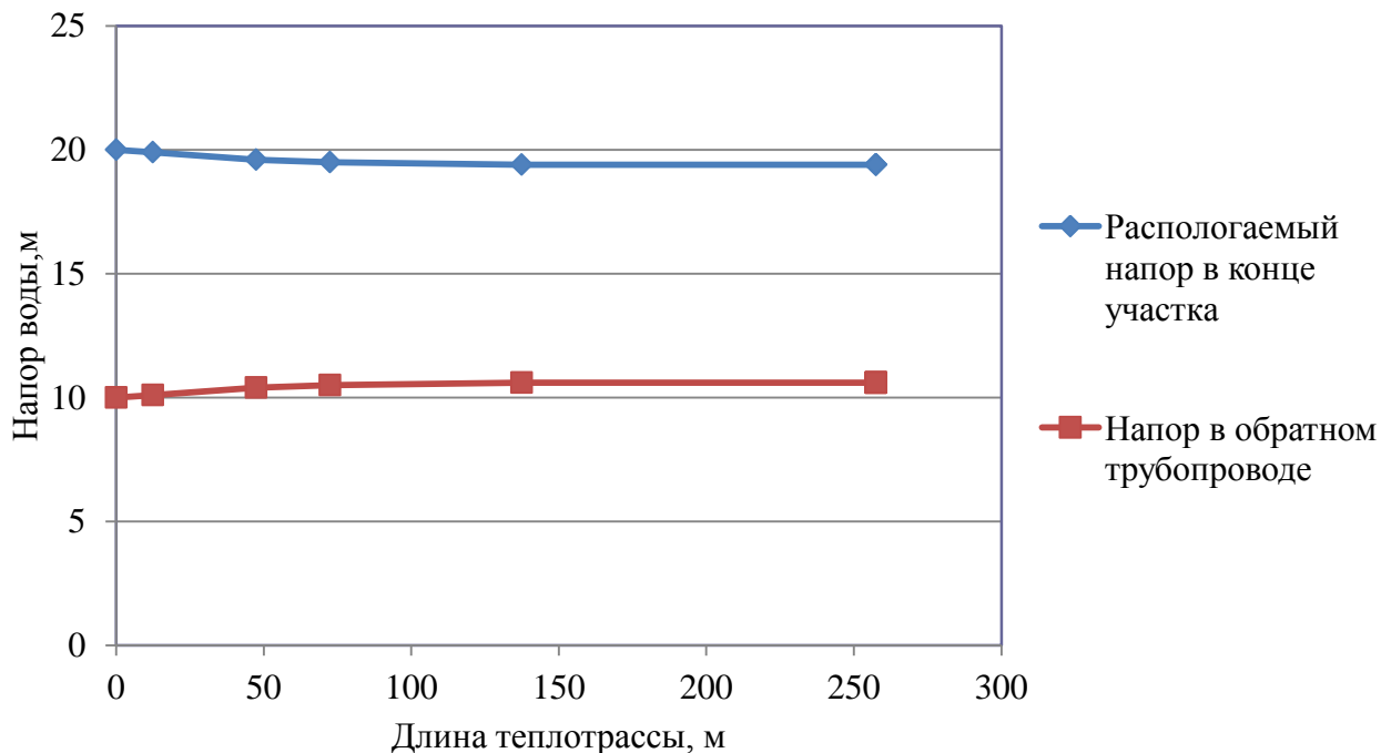
Рисунок 2.7 – Пьезометрический график тепловой сети центральной котельной с. Новодостовалово
