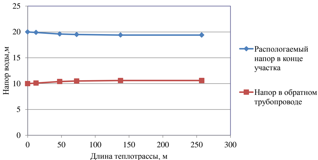
Рисунок 2.5 – Пьезометрический график тепловой сети центральной котельной с. Новодостовалово
