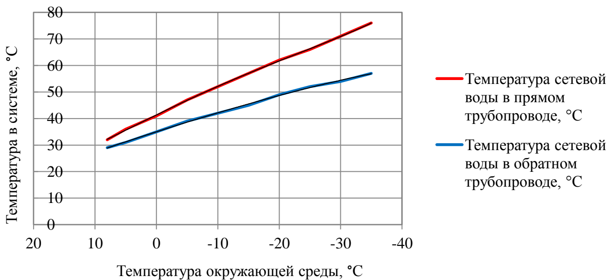
Рисунок 2.4 – График изменения температур теплоносителя 80-60°C
