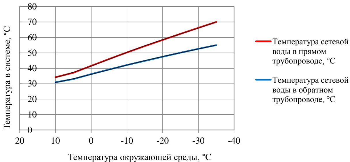
Рисунок 2.3 – График изменения температур теплоносителя 70-55°C
