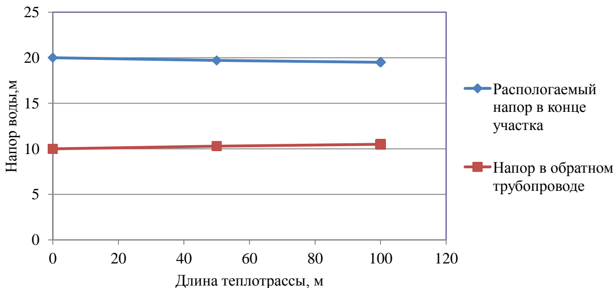
Рисунок 2.8 – Пьезометрический график тепловой сети школьной котельной с. Романовское
