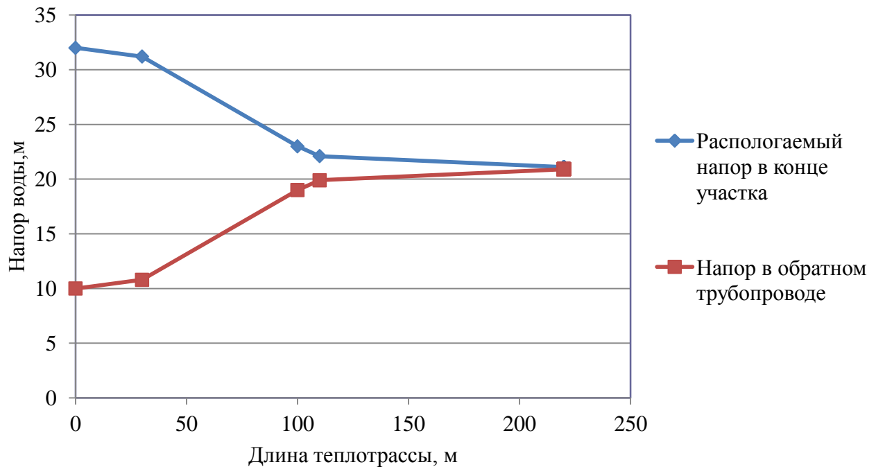
Рисунок 2.5 – Пьезометрический график тепловой сети котельной с. Скопино
