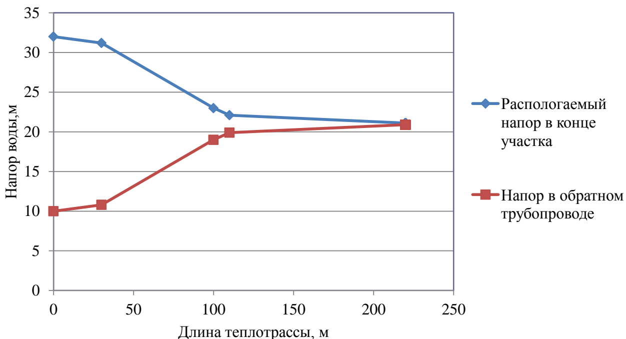
Рисунок 2.4 – Пьезометрический график тепловой сети котельной с. Скопино
