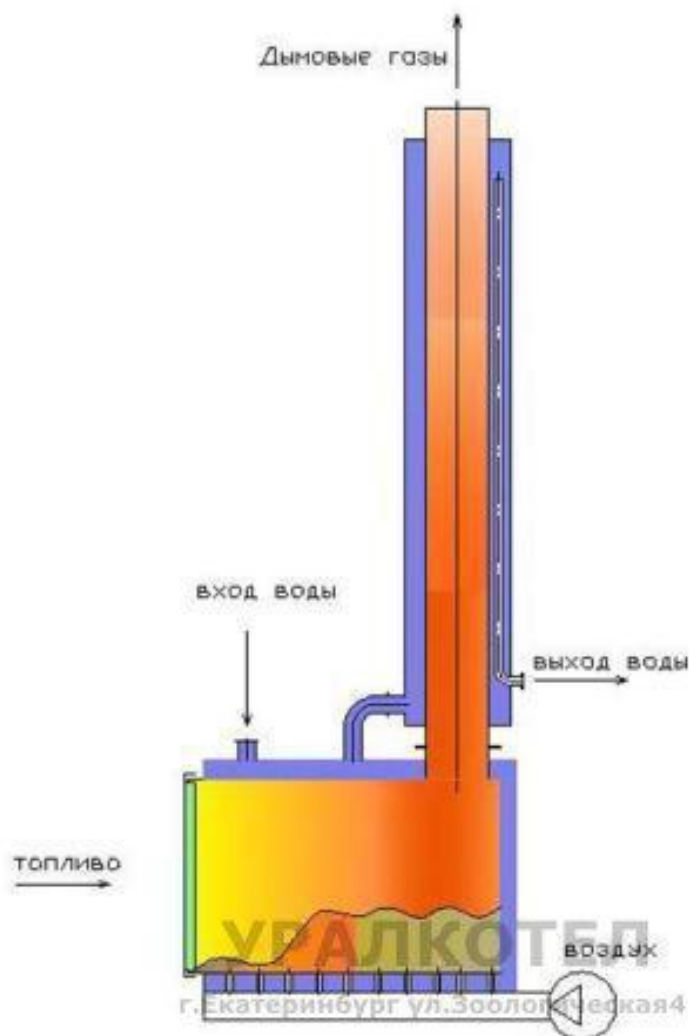
Рисунок 2.1 – Принципиальная схема котла КВРСрд-0,5
